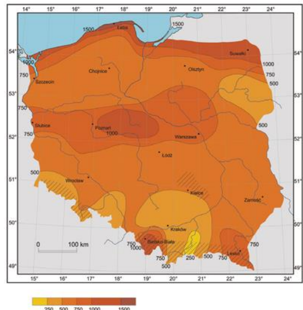
Rys. 19 Teoretyczna gęstość mocy wiatru (wyrażona w kWh/(m 2 *a)) na wysokości 10 m n.p.g. w terenie otwartym o niskiej szorstkości.
